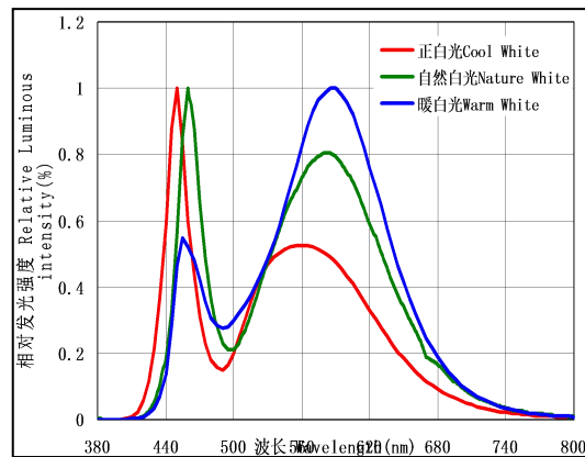
光谱特性图
