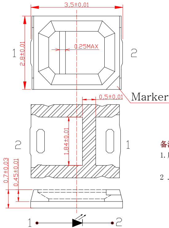
封装尺寸 Package Dimensions
