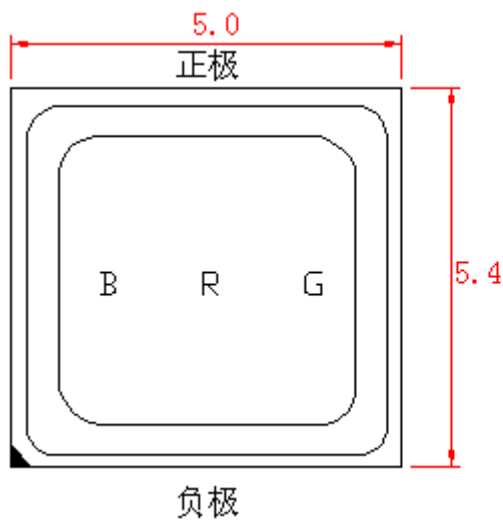
封装尺寸 Package Dimensions
