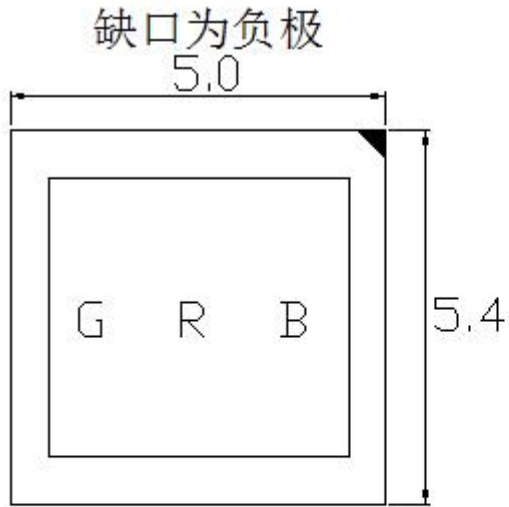
封装尺寸 Package Dimensions
